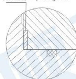
中法兰防火结构 Middle flange fireproof structure
