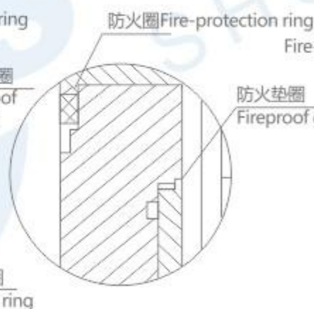
中法兰防火结构 Middle flange fireproof structure
