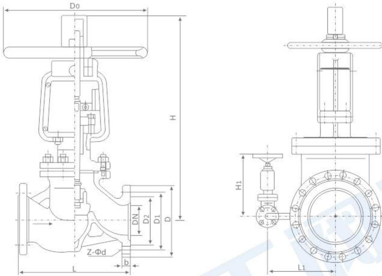
主要外形及和连接尺寸 Main external and connection dimension JB/T79.2 单位Unit:mm
